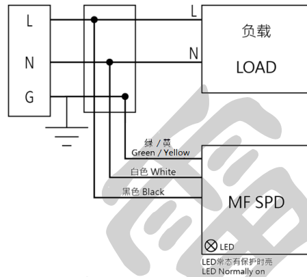
并联接法 Parallel Connection
